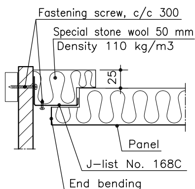
DET. 3 (ALT.2)
