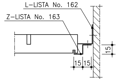
Säädettävä asennustapa
