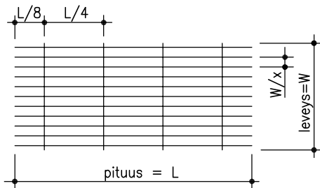
Ritiläelementin mitoitusesimerkki
