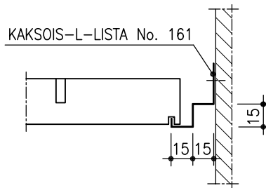
Kiinteä asennus
