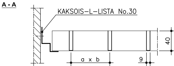
VALAISIMEN ASENNUSLAATIKKO
