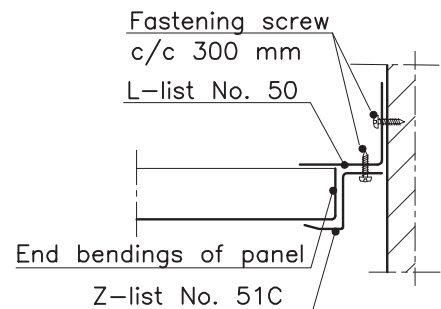
DET. 2 (ALT. 2)
