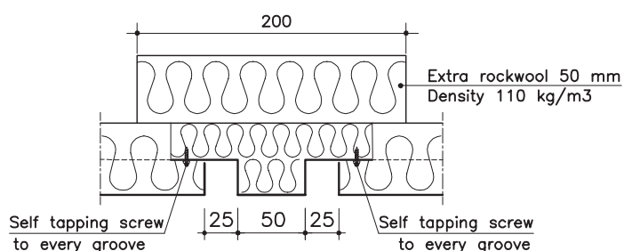
D-D (A)
