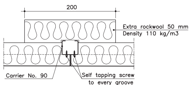
D-D (B)
